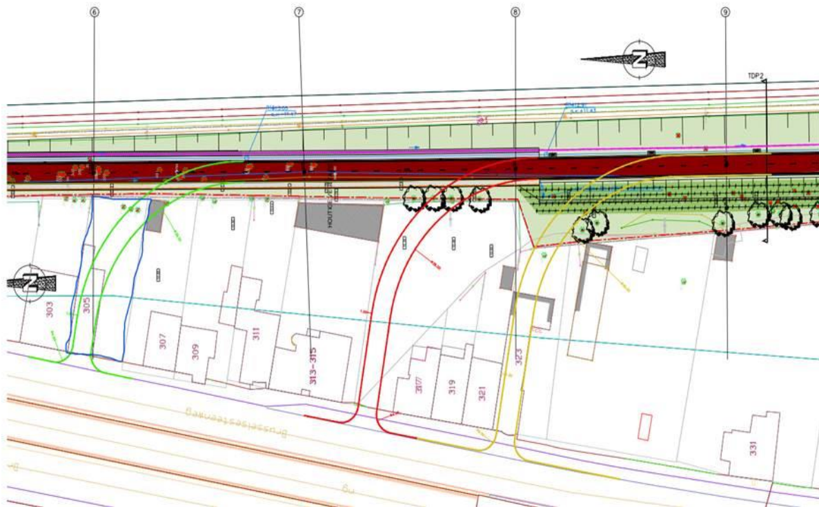
Figuur 2: intekening fietsostrade-tracé op varianten
